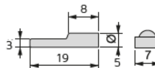
MENSOLINE IN FERRO CON O-RING IN GOMMA PERNO MM 5
