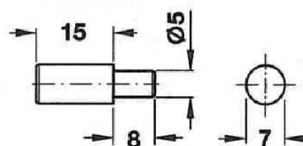
ART. 71 MENSOLINE FERRO NICHELATO A PALETTA PERNO MM 5
