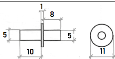
ART. 50623 MENSOLINE DOPPIE FERRO ZINCATO
